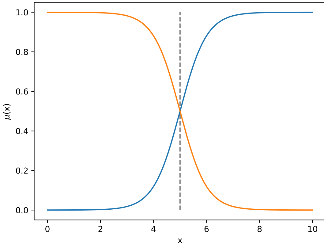
Sigmoid(a=5, b=-2)
