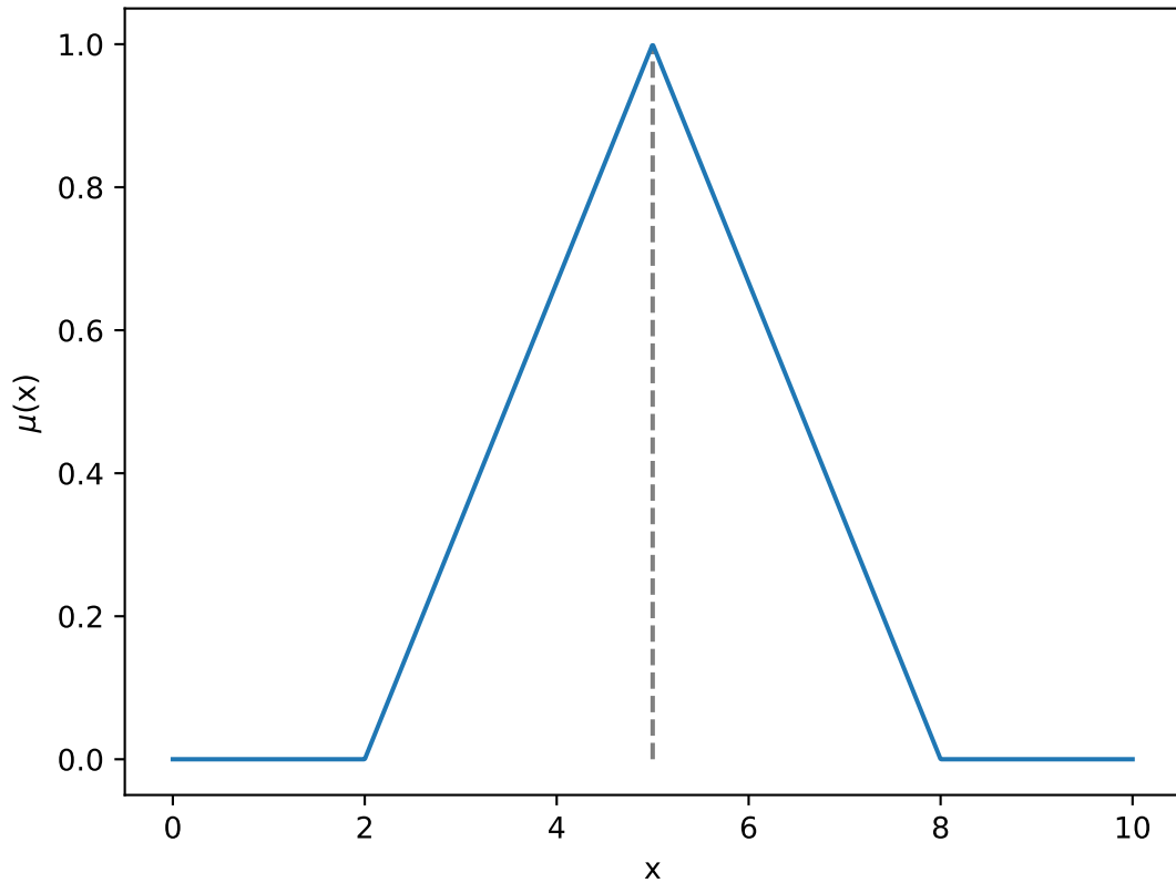
Triangle(a=2, b=5, c=8)
